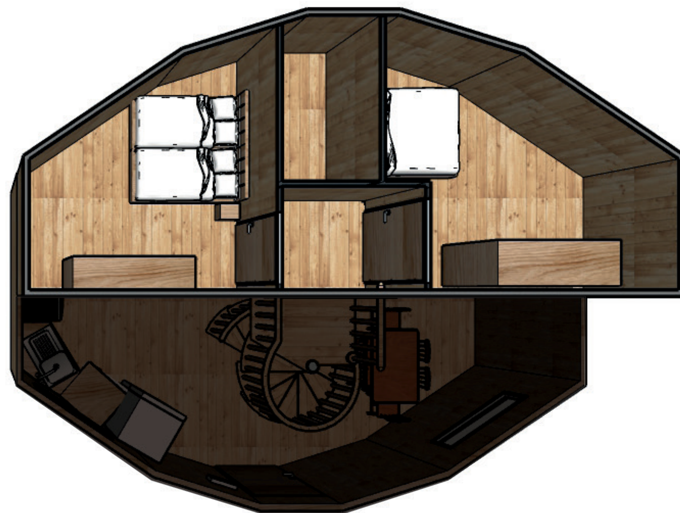
Maison Poule 4/6 personnes environ 47m 2
