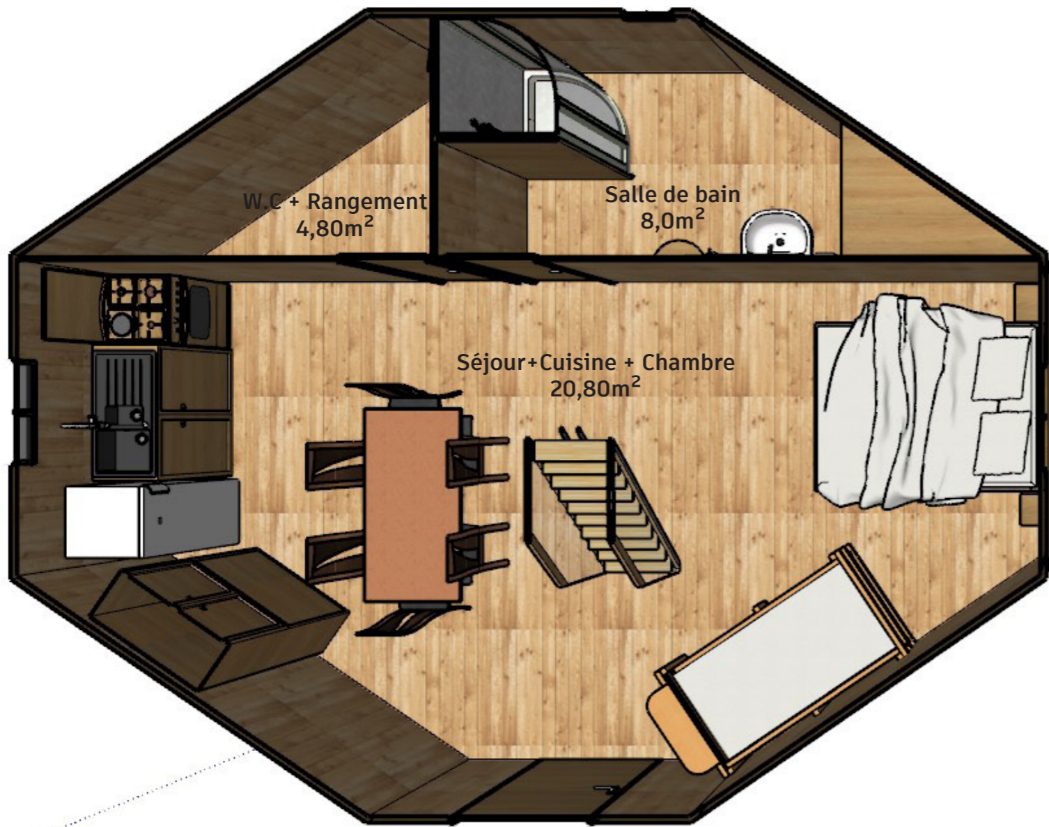
PLAN Rez-De-Chaussée
